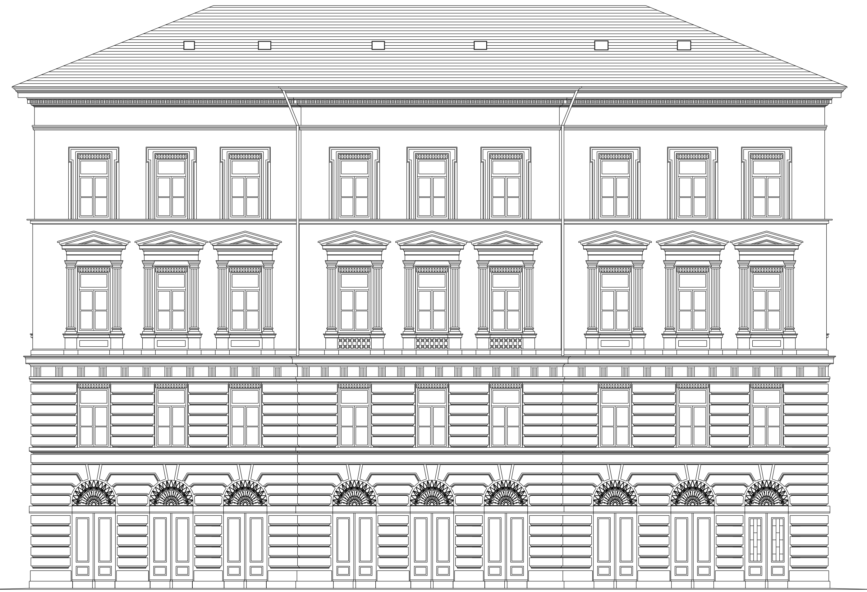
PROSPETTO SU VIA DEL TEATRO ROMANO
